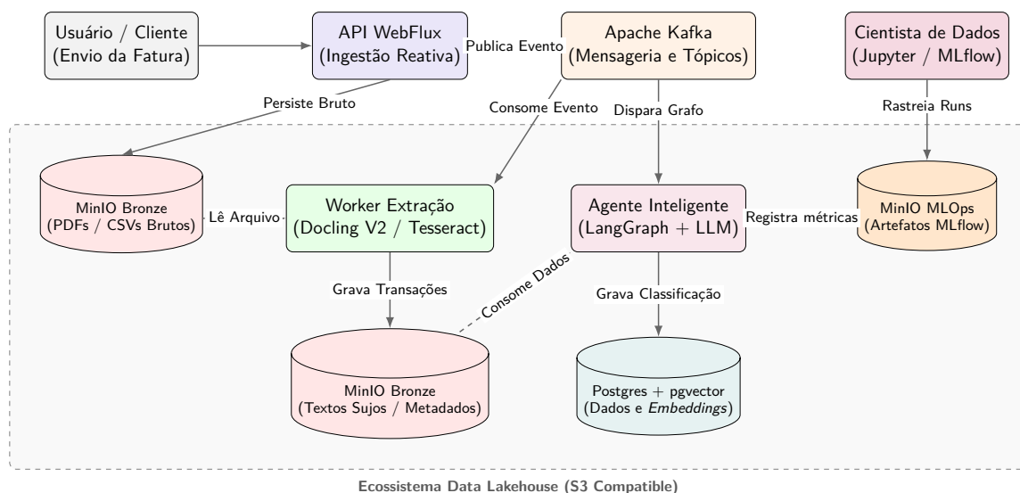
Figura 1 – Arquitetura de Data Lakehouse orientada a eventos com MLOps e agentes de IA.
